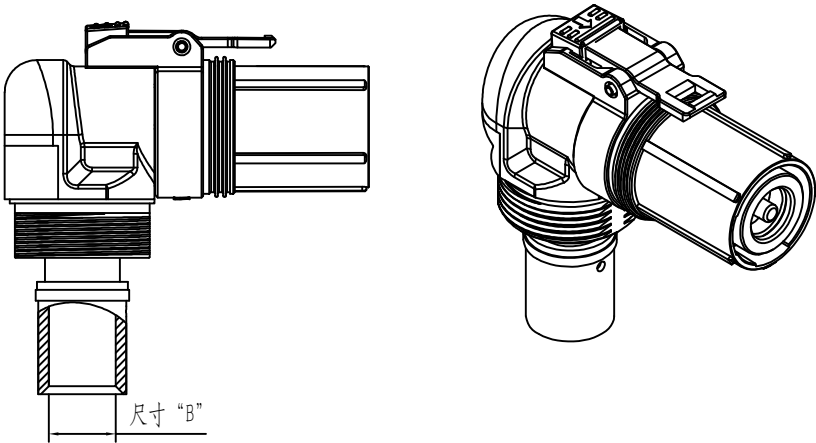
插头主体
